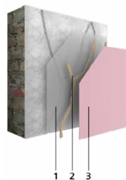
1 Grundbeschichtung 2 Rissverfüllung 3 Schlussbeschichtung
